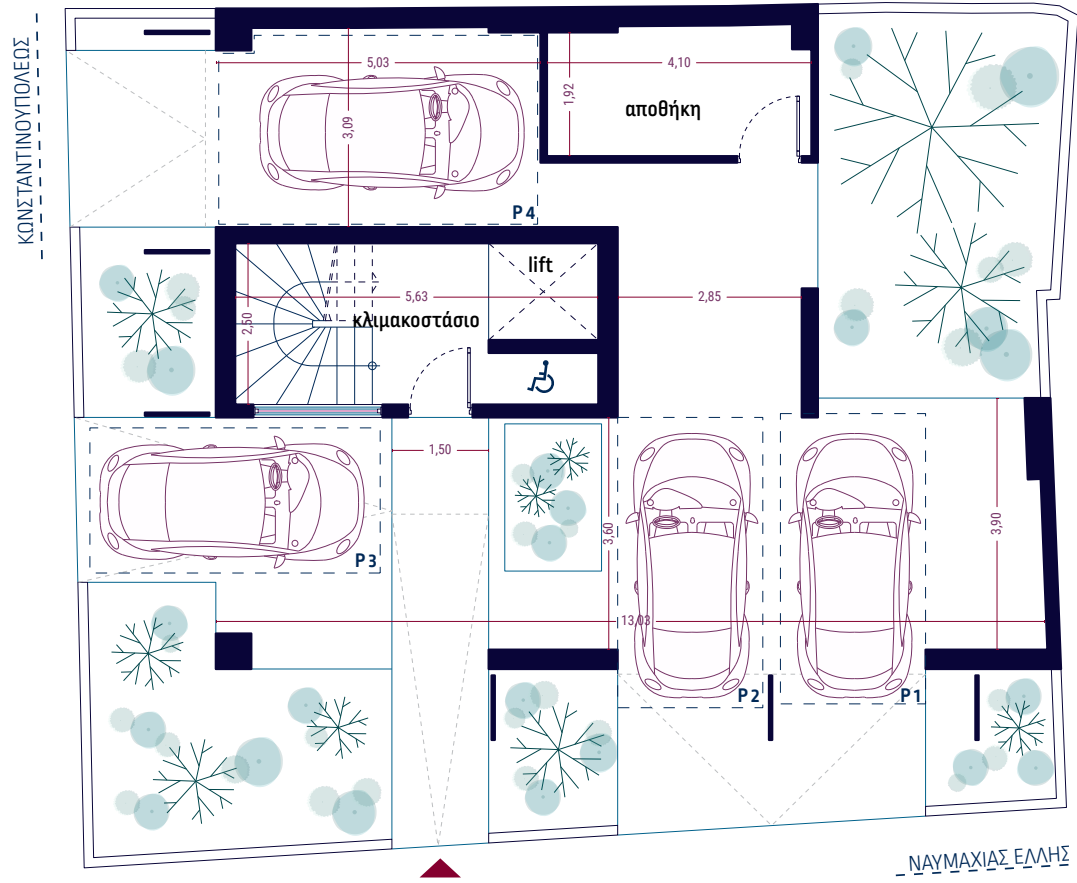
ΚΑΤΟΨΗ PILOTIS
